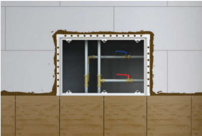
PVC rámeček, magnety, pozinkovaný plech
