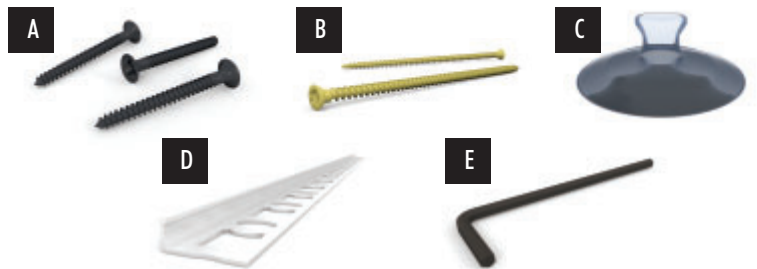
[A] šrouby do sádrokartonu | [B] turbošrouby | [C] přísavka | [D] PVC lišta | [E] imbus klíč
